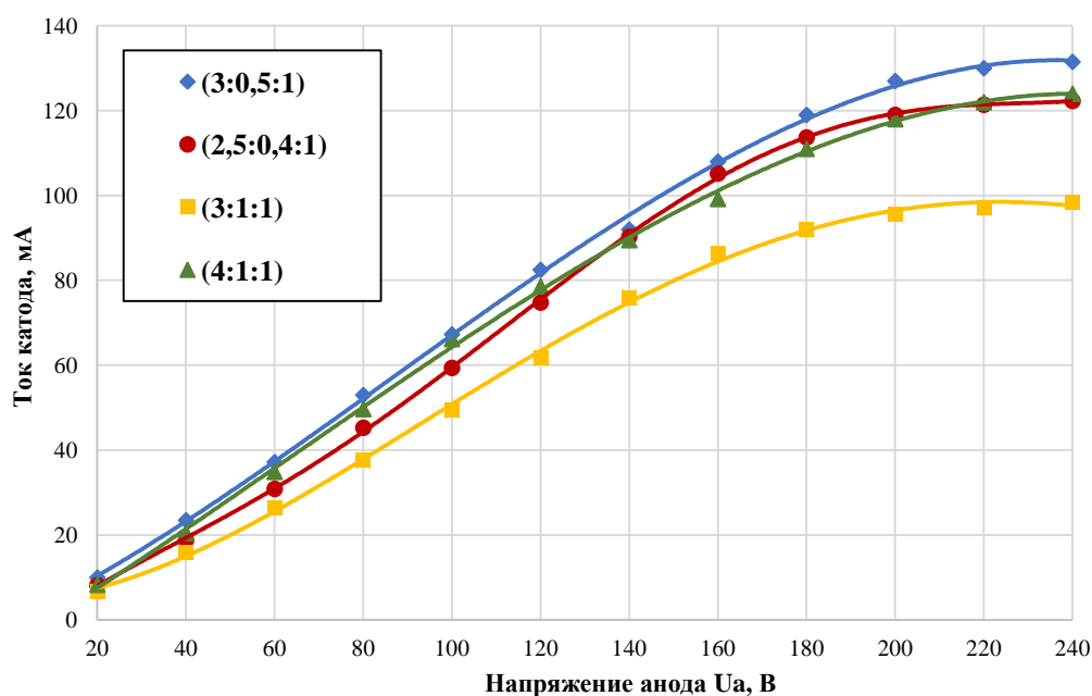
Рис. 3. Семейство ВАХ при температуре T_{ист.} = 1120^{\circ}\text{C}
