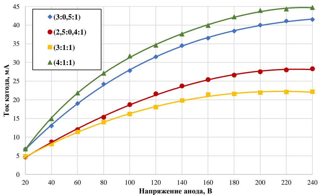
Рис. 2. Семейство ВАХ при температуре T_{\text{ист.}} = 915^\circ\text{C}
